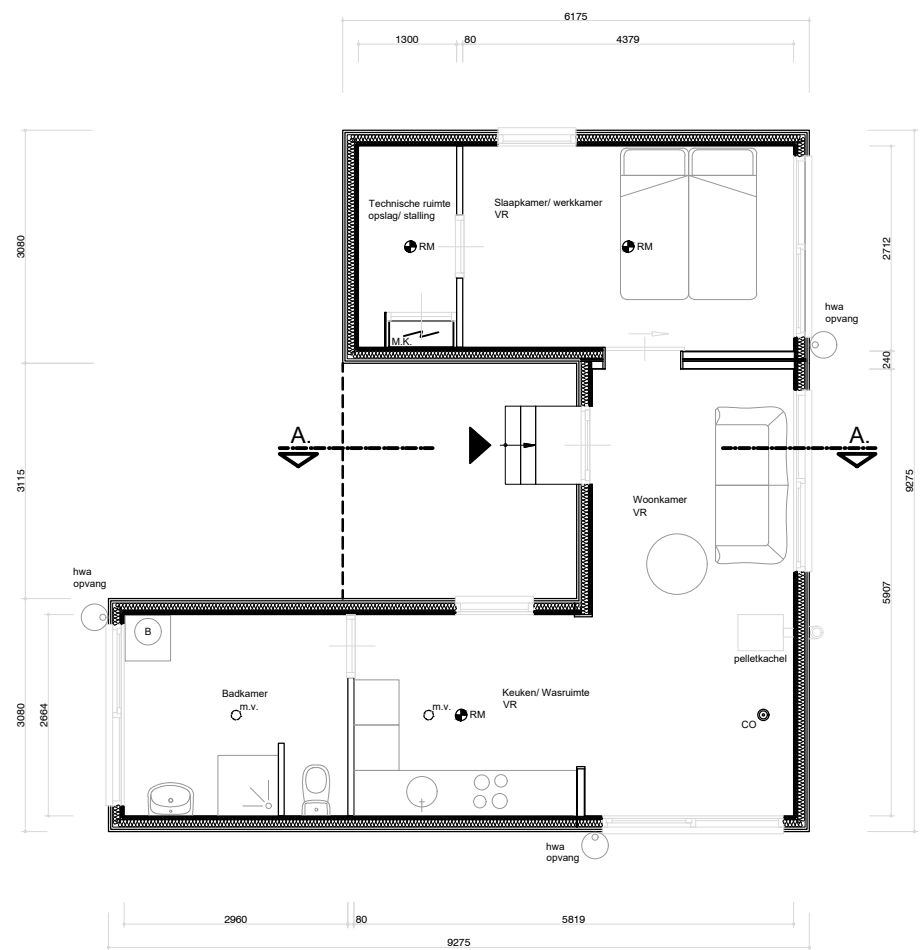
Plattegrond
