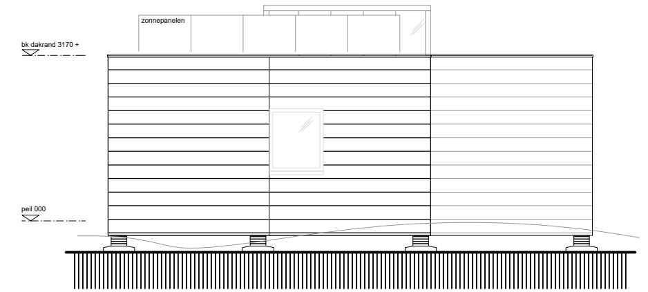
Gevel noord
