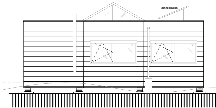
Gevel oost
