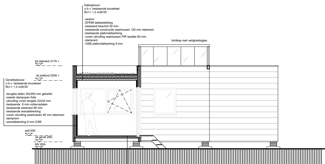
Doorsnede A-A
