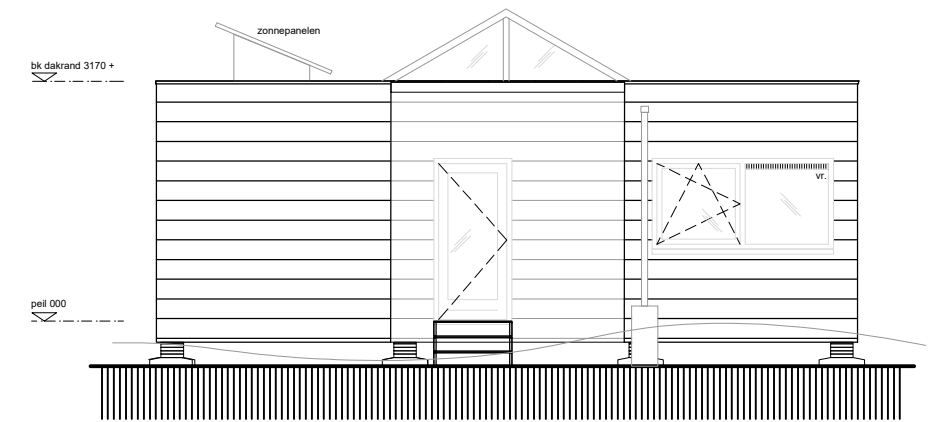
Gevel west
